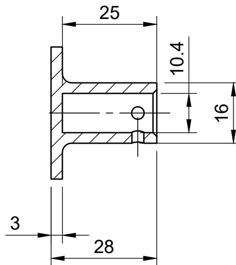
A-A (1:1)
